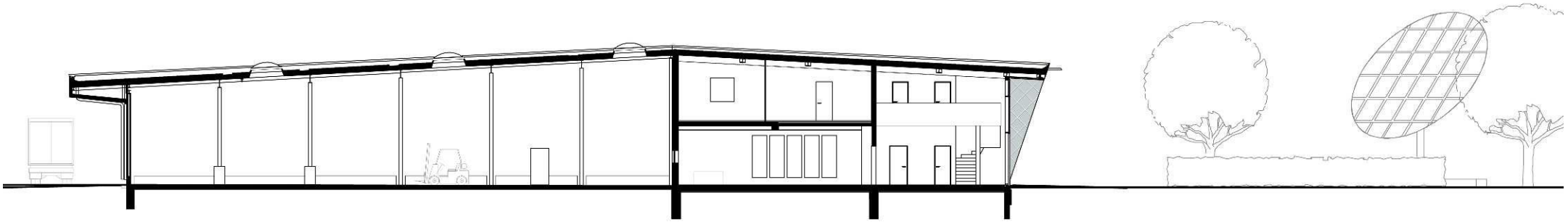
Schnitt A-A
